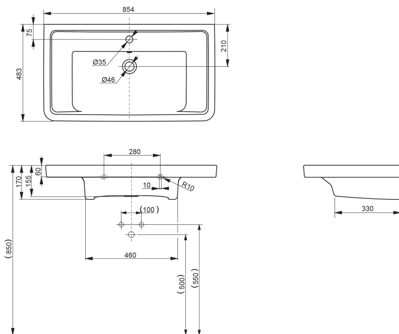
LT137CW
